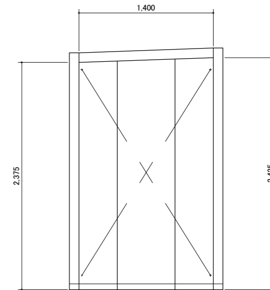
B内視図
