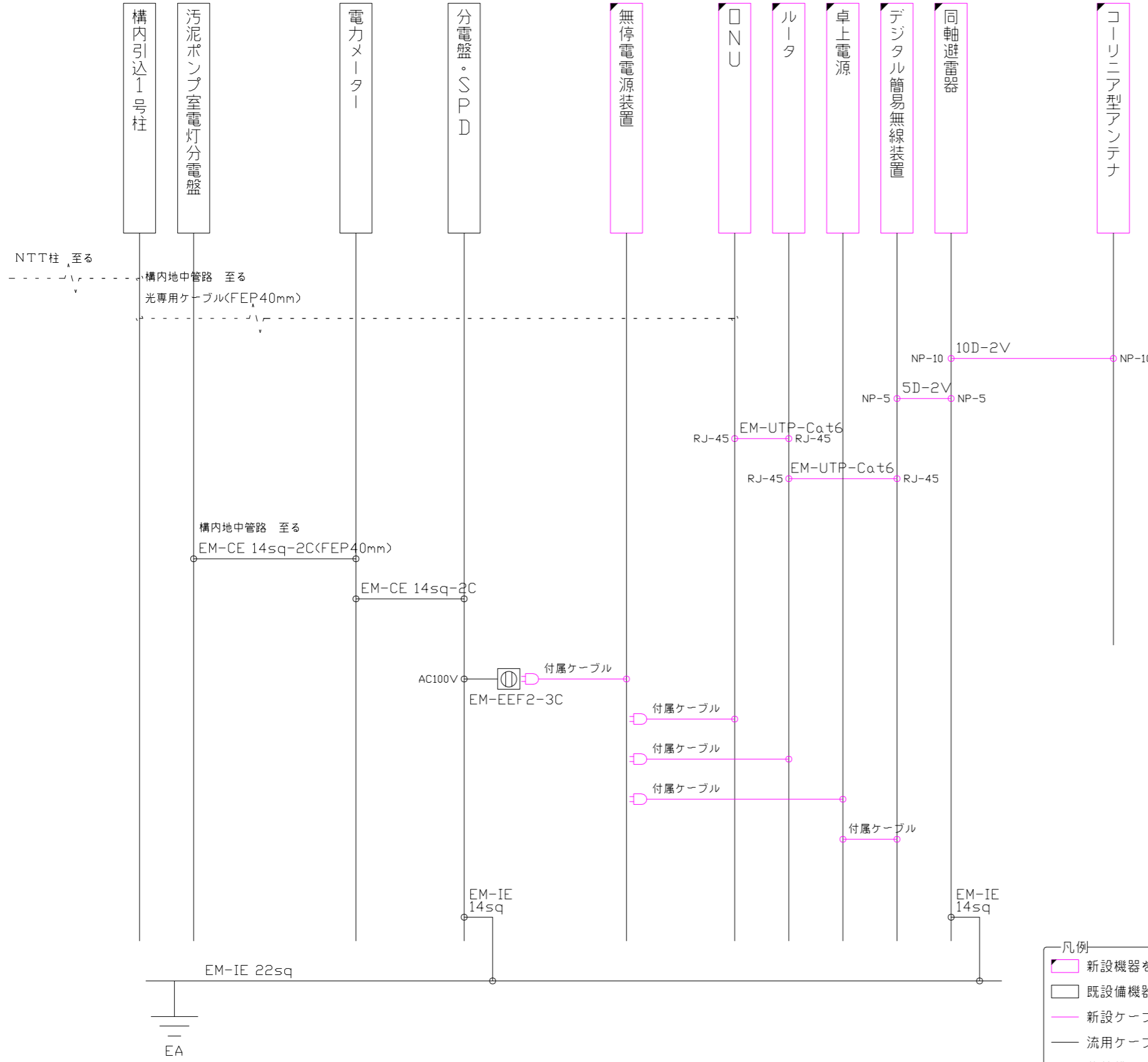
ケーブル系統図
