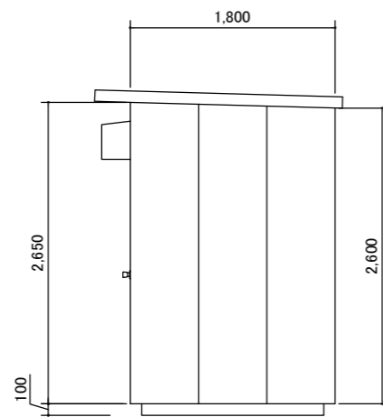
B 立面図
