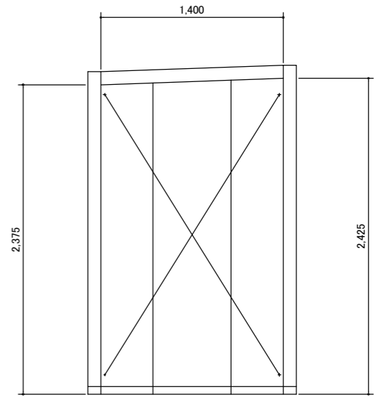
B 内視図
