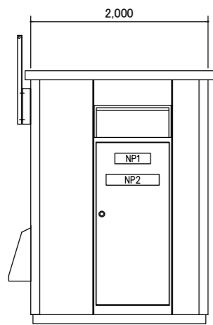
A 立面図
