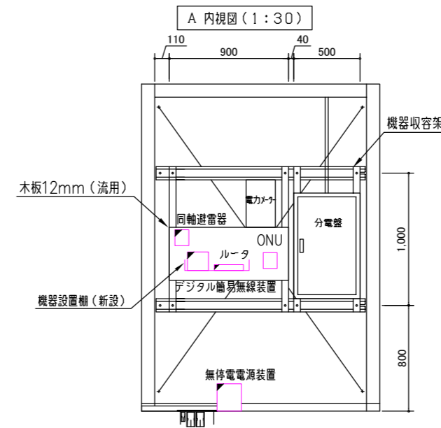
C 内視図
