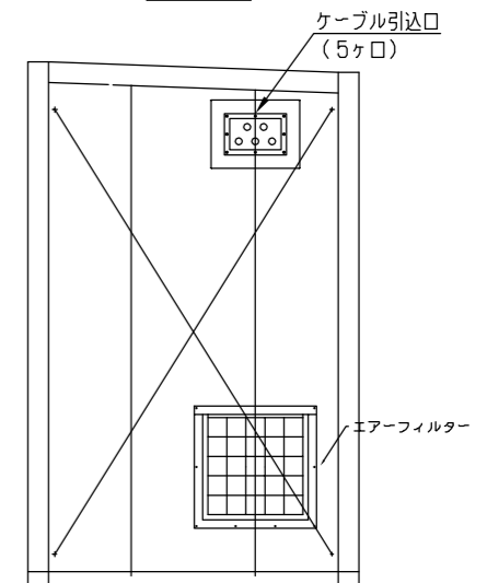
B 内視図
