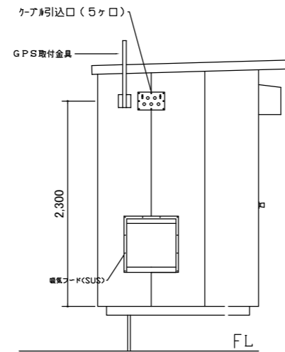
D 立面図
