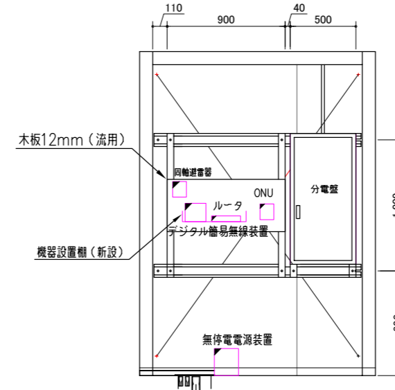
A内視図
