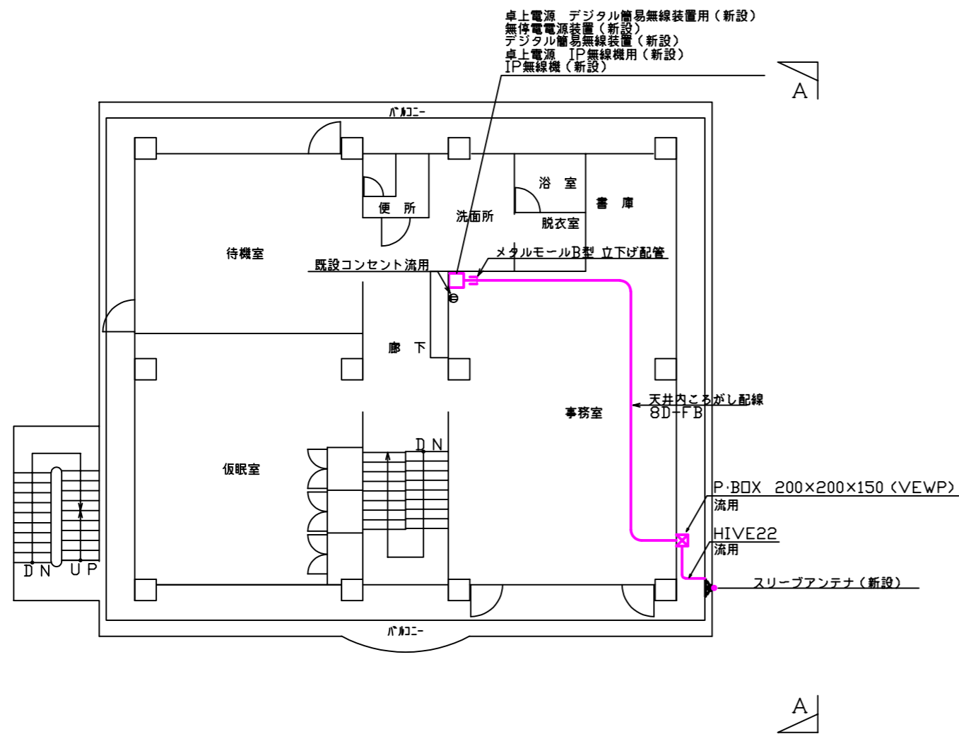
2階平面図 S=1/150
