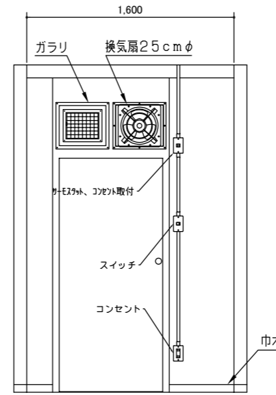
A 内視図 (1:30)
