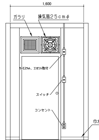
A内視図
