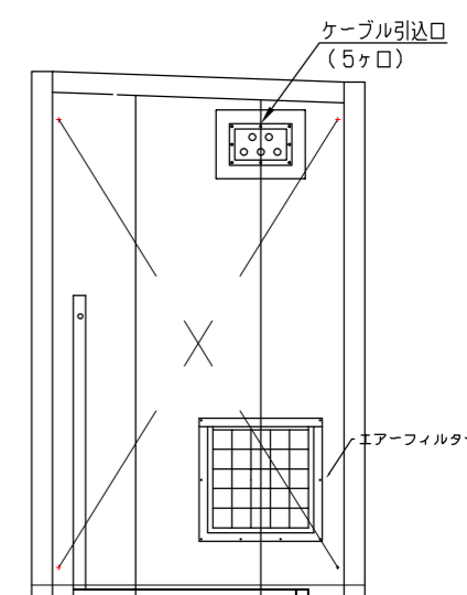
B内視図
