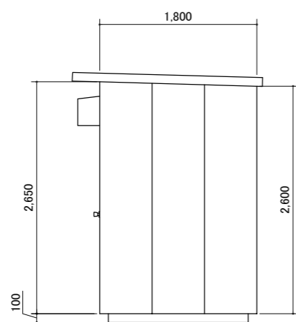
B立面図
